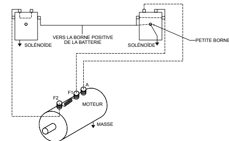
FIGURE 3 CONNEXIONS DU SOLENOÏDE AU MOTEUR
