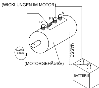
ABBILDUNG 2 MOTOR – DREHUNG NACH LINKS
