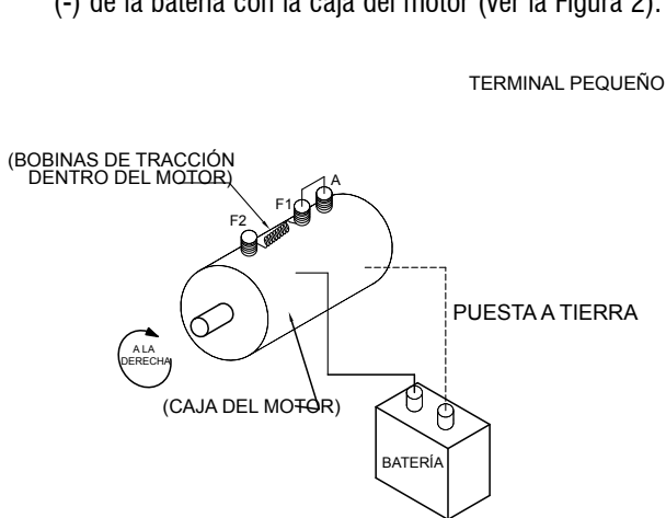
FIGURA 1 MOTOR - GIRO A LA DERECHA
