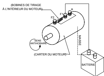
FIGURE 2 MOTEUR : ROTATION SENS ANTIHORAIRE
