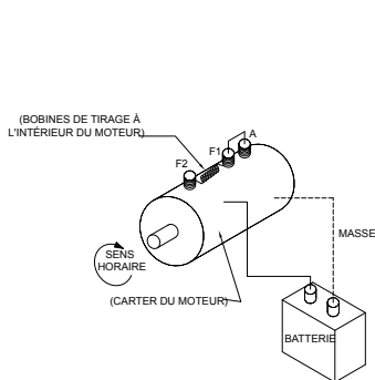
FIGURE 1 MOTEUR : ROTATION SENS HORAIRE
