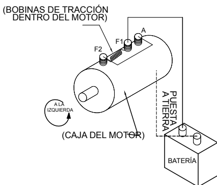
FIGURA 1 MOTOR - GIRO A LA IZQUIERDA
